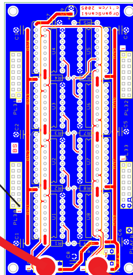
OrganScan61- Platinen Obermanual Unterste Taste
